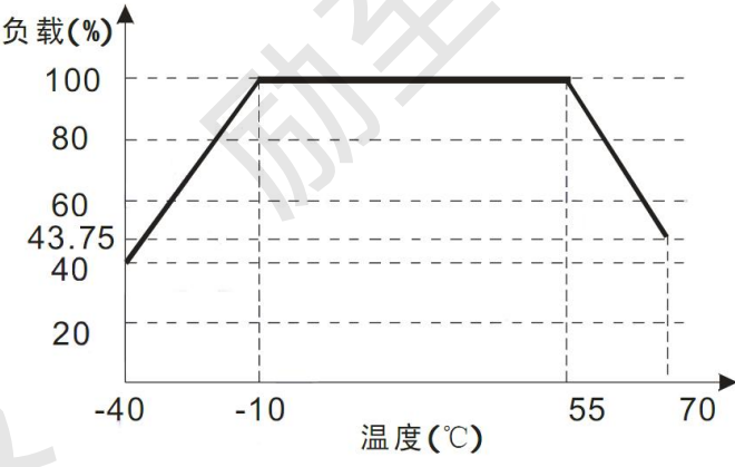
温度与负载关系图
