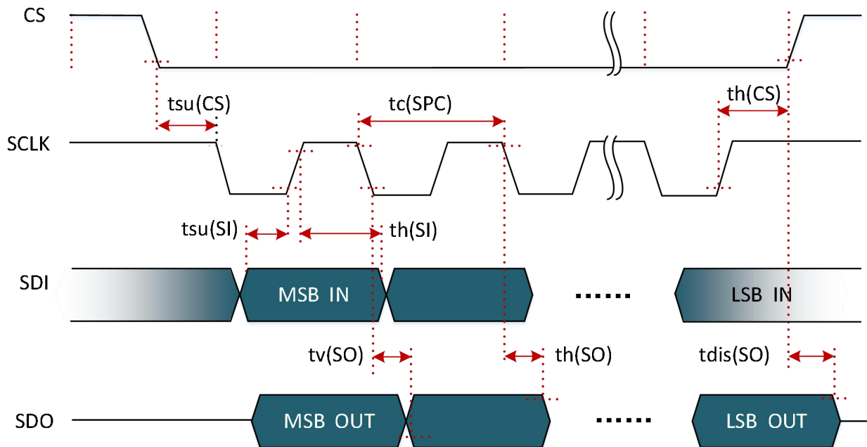
图 12-1 SPI 时序图
