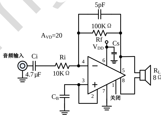
图2、高增益电路
