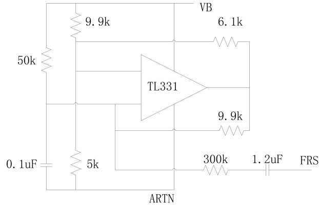
图29 频率抖动
