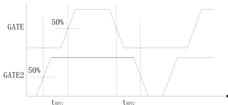
图 2 GATE和GATE2时间和相位
