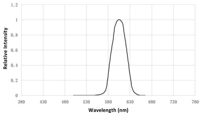
光谱分布特性曲线 Spectrum Distribution ( T_a=25^{\circ}\text{C} )
