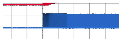
图 16. PFM 模式 满载 EN 关机
