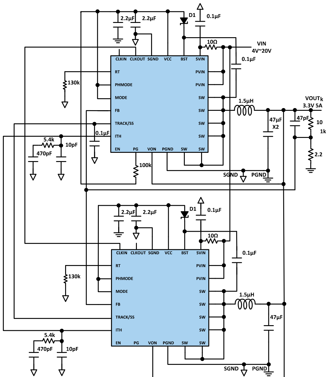
图 3.3V 双相单路 10A 输出降压电路
