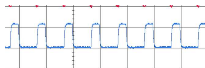
图 14. PFM 模式满载 EN 开机
