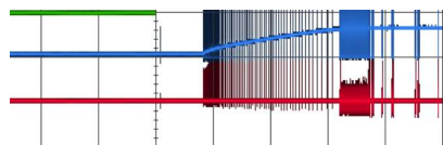
图 15. PFM 模式空载 EN 关机
