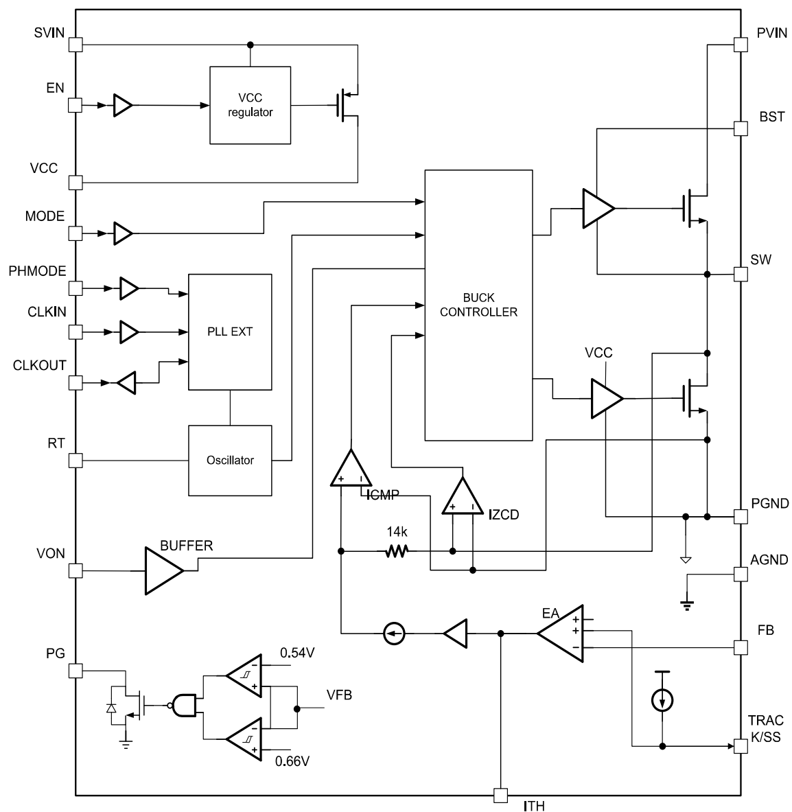
图 4 内部功能框图
