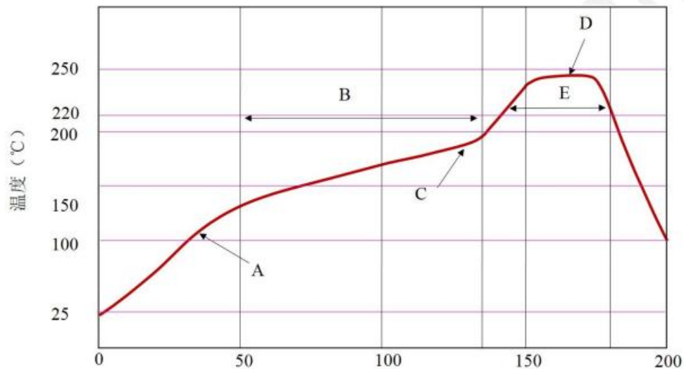
图 7 炉温曲线
