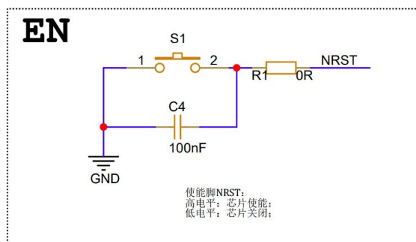
图 4 按键复位参考设计
