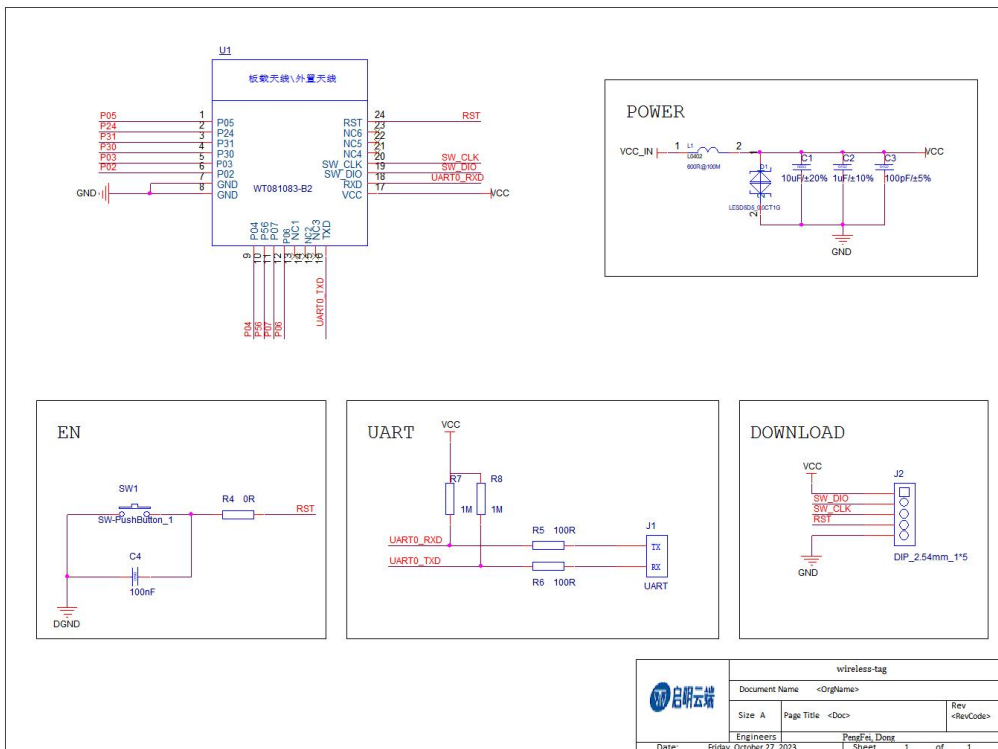
图 7 应用模组外围设计原理图
