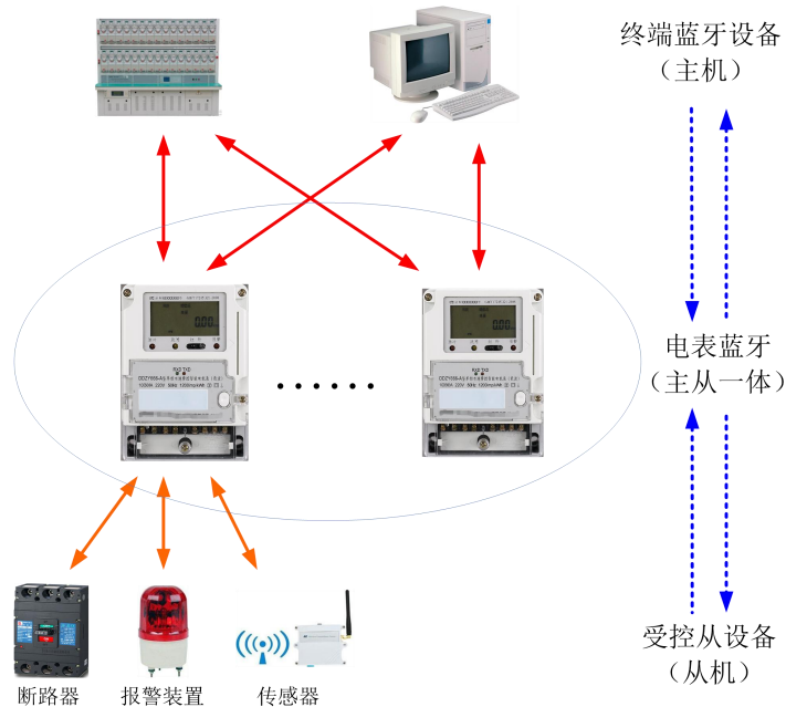
图 9 蓝牙网络拓扑图
