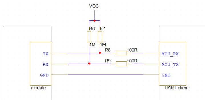
图 5 串口连接参考设计
