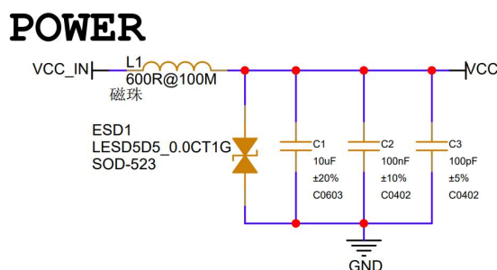
图 3 推荐电源设计
