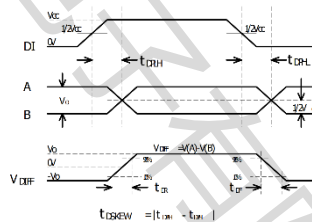
图 5 驱动器传输延时
