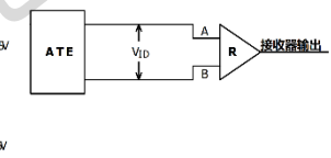
图 9 接收器传输延时测试电
