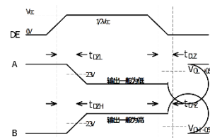
图 6 驱动器使能/关断时序
