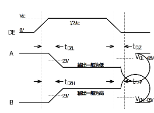
图 6 驱动器使能/关断时序
