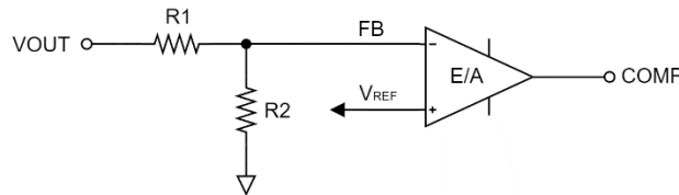
图 7.1 设置输出电压
