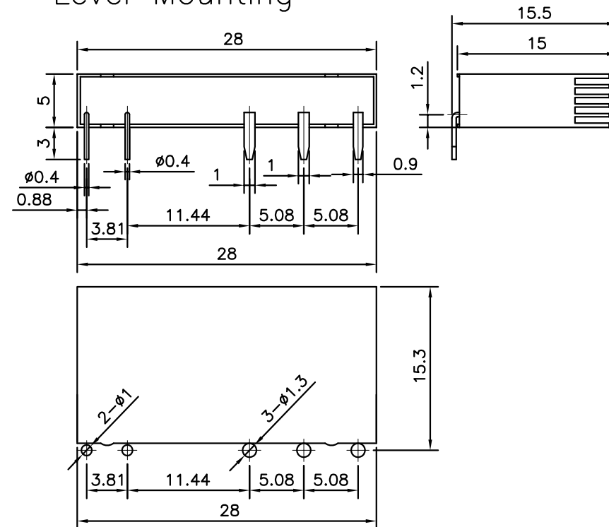
P.C.B LAYOUT
