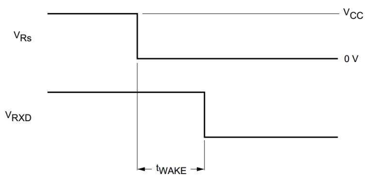
图 5 从待机状态唤醒时序图
