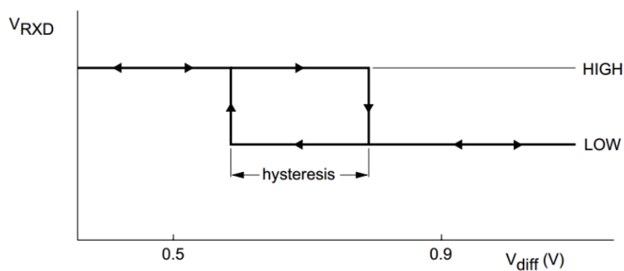
图 4 迟滞
