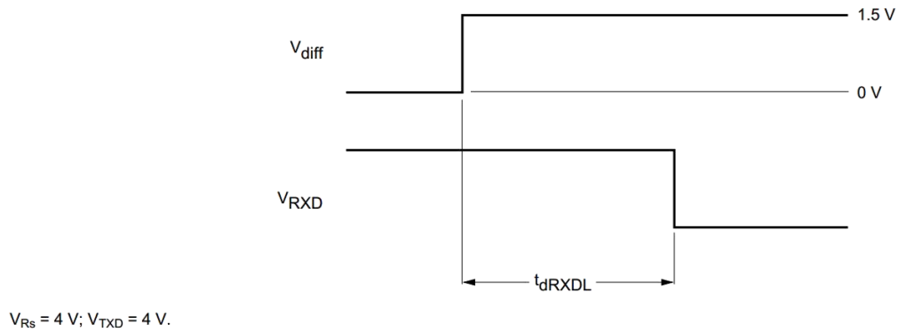
图 6 总线显性到 RXD 输出低时序图
