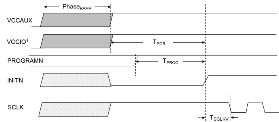
图 3-1-2 器件上电时序图
