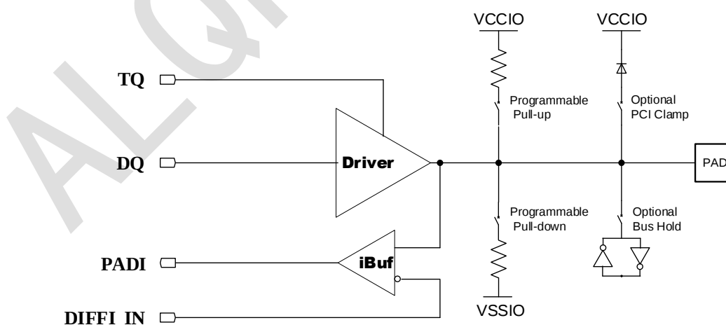
图 2-8- 1 基本 IOBE 框图
