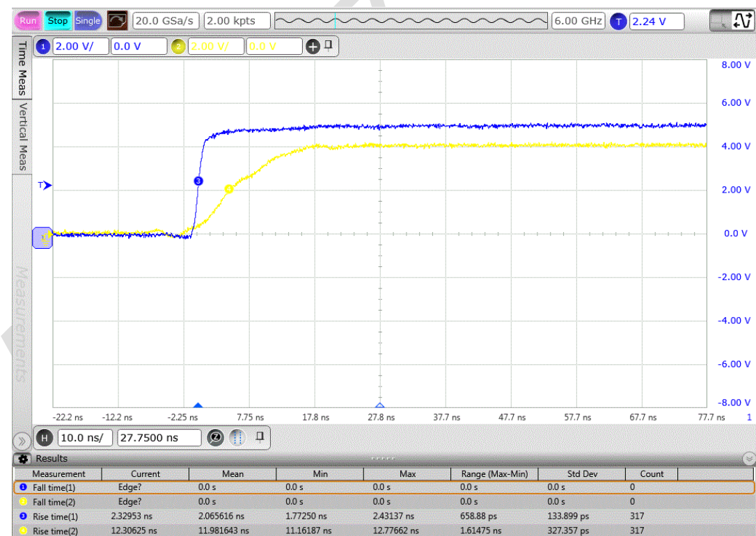
图 2-8- 7 5V 输入驱动 ELF2 器件接收端波形 @R=330 0hm
