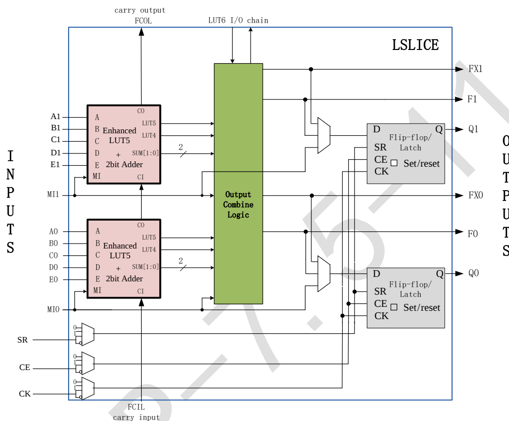
图 2-1- 3 LSLICE 结构图
