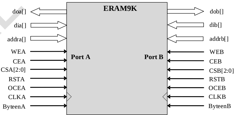
图 2-3- 9 9 位宽≤9 位时 A/B 双口 RAM
