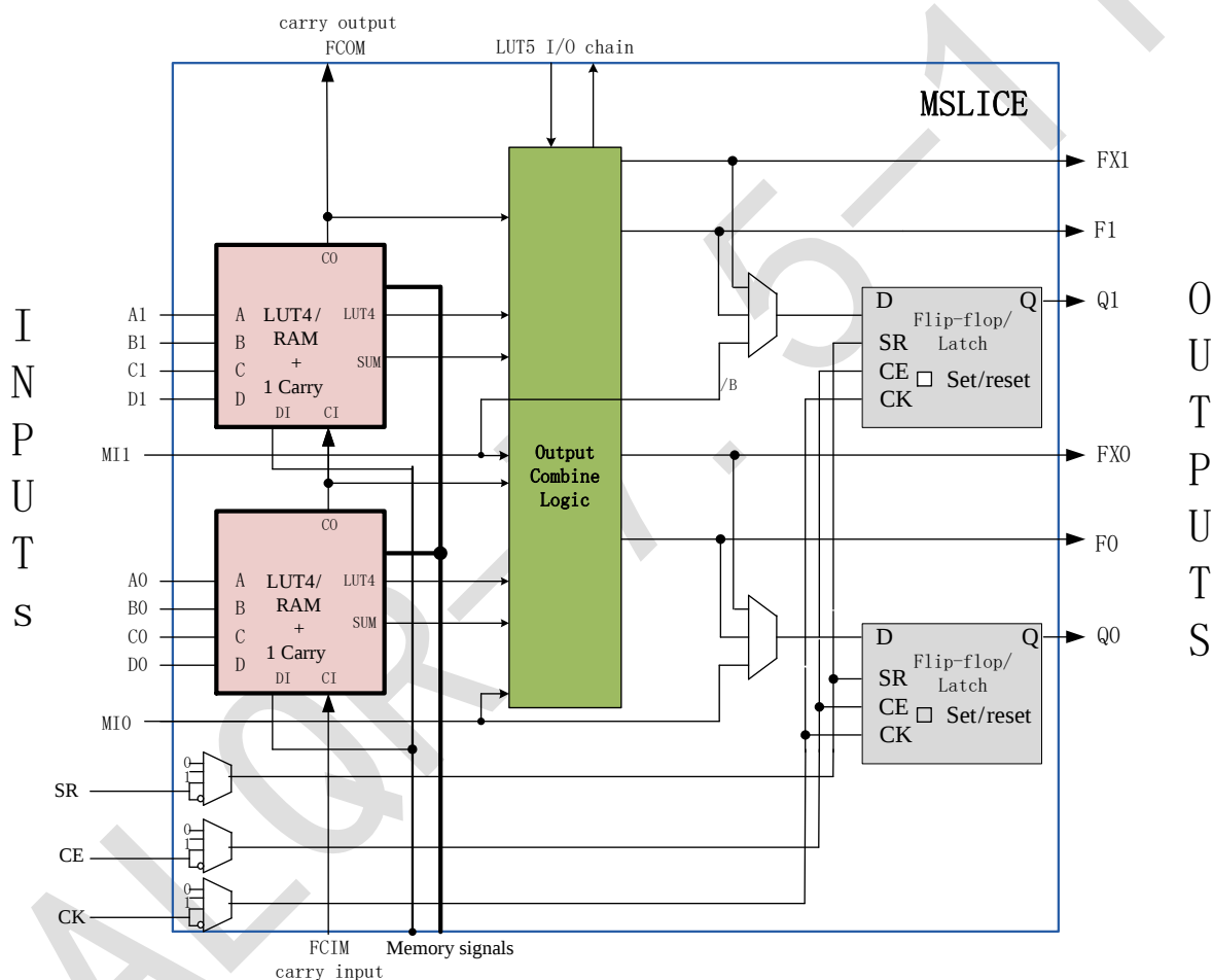
图 2-1- 2 MSLICE 结构图
