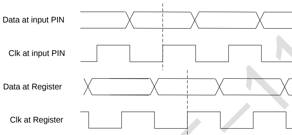
图 2-5- 4 源同步模式
