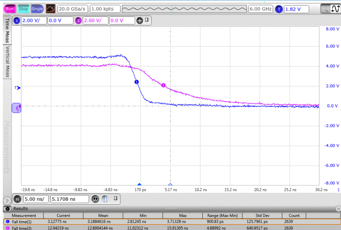
图 2-8- 7 5V 输入驱动 ELF2 器件接收端波形 @R=330 0hm
