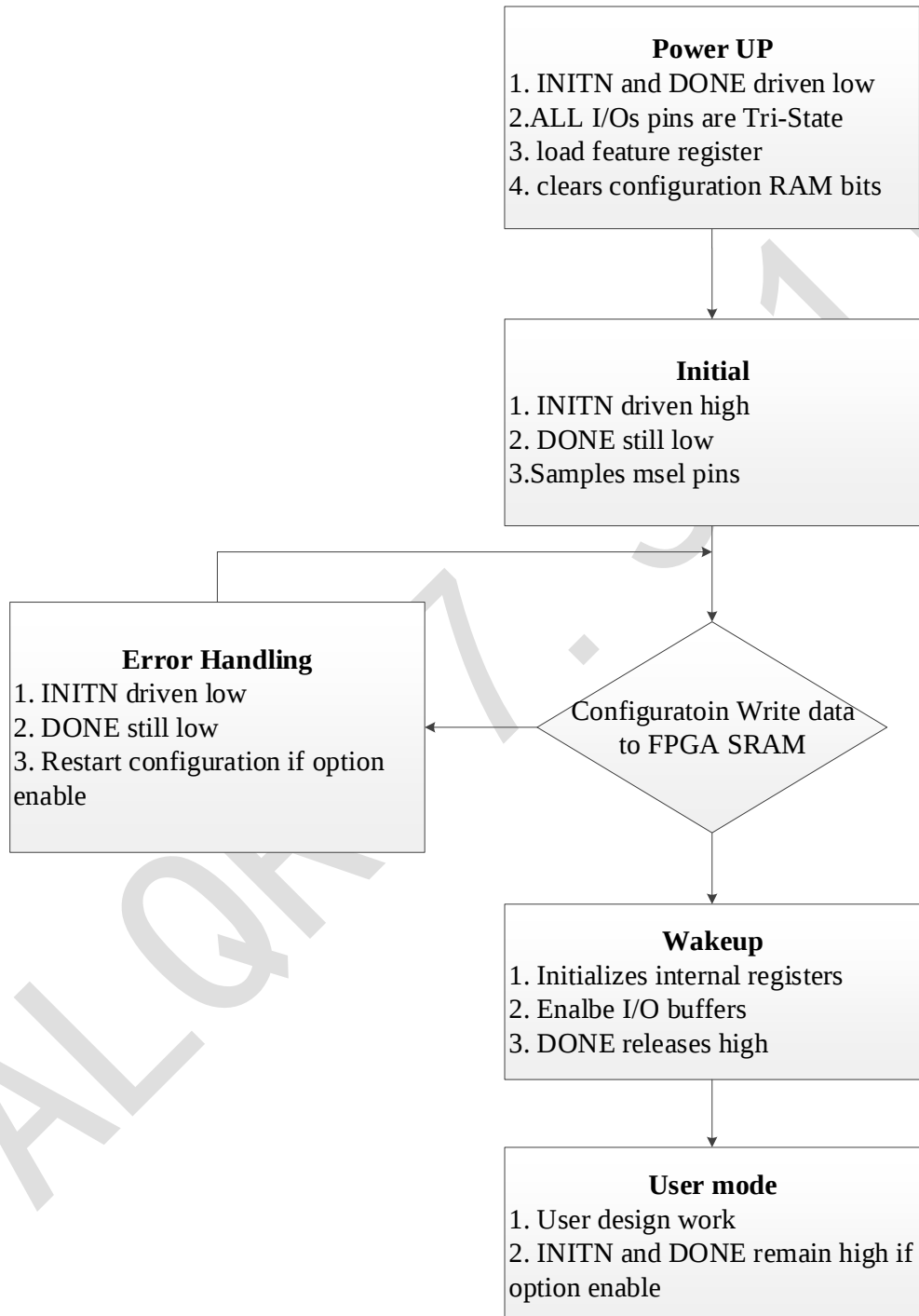
图 2-9- 1 ELF2 MSPI 配置流程
