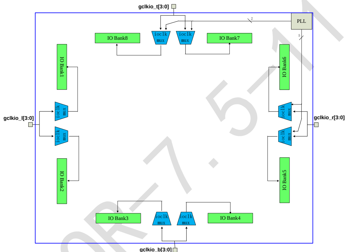
图 2-4- 4 IOCLK 架构图
