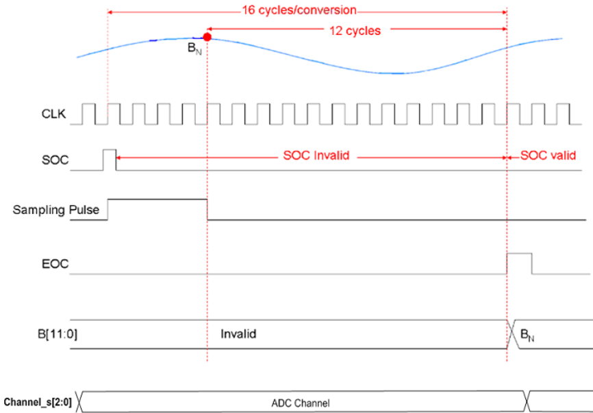
图 2-10- 1 ELF2 ADC 采样控制时序
