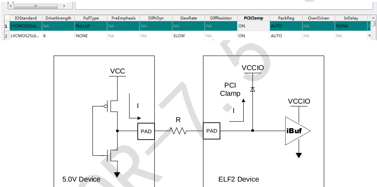
图 2-8-6 5V 输入驱动 ELF2 器件
