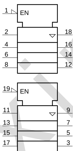
图 2 IEC 逻辑符号
