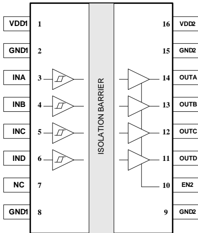
图 1. CMT8040x 管脚
