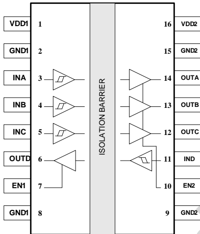
图 2. CMT8041x 管脚
