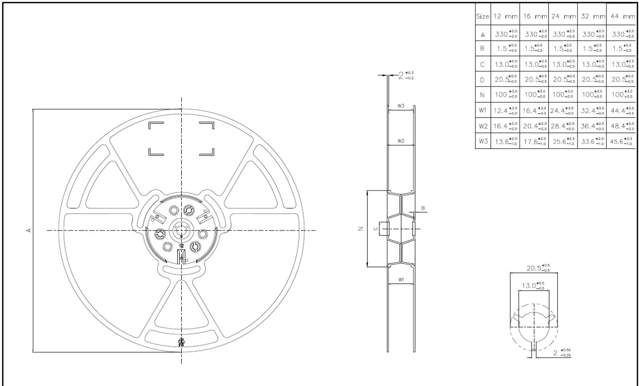
图 15. CMT804X WB SOIC-16 卷带信息
