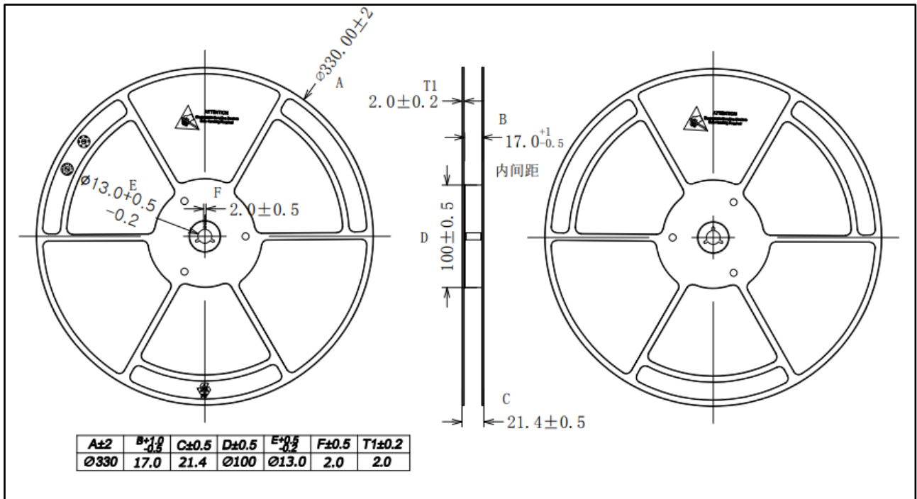
图 17. CMT804X NB SOIC-16 卷带信息
