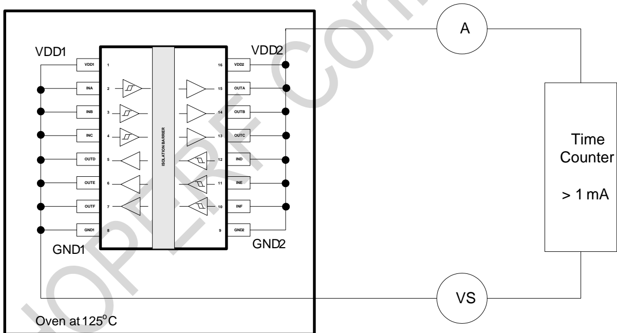
图 9.绝缘寿命测试方式
