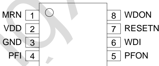
图 2、引脚图
