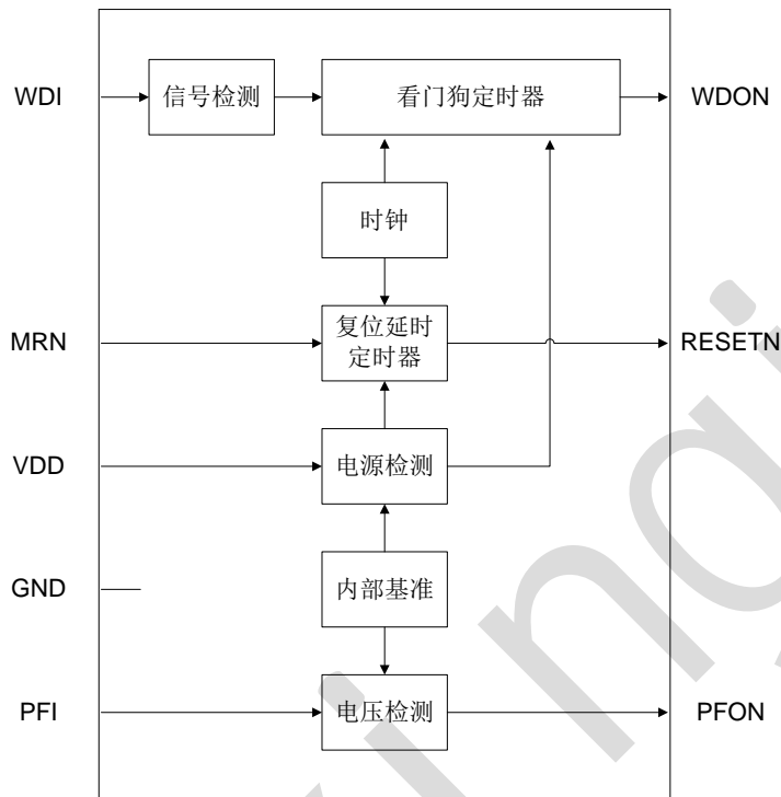
图 1、功能框图
