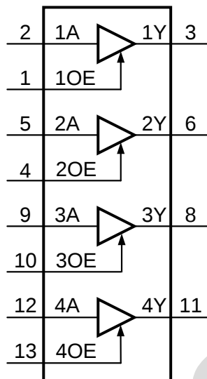
图 1 逻辑符号
