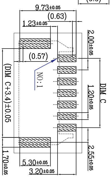
适用线路板 (PCB LAYOUT)
