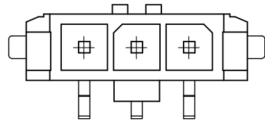
3PIN
