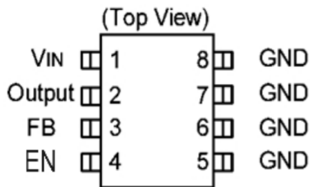
SOP8
