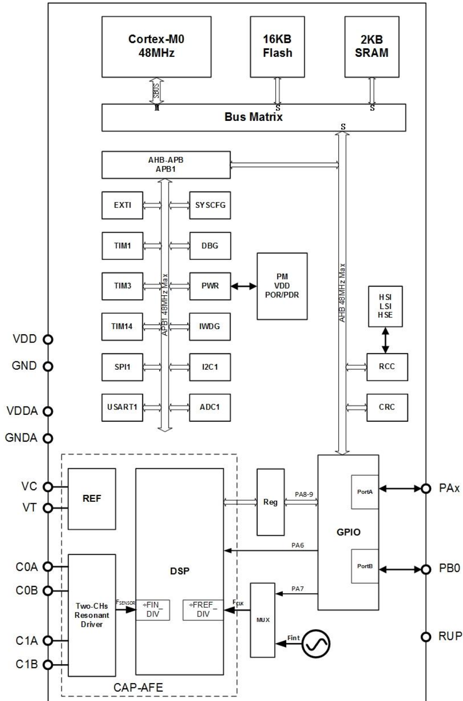
图 6.1 系统框图
