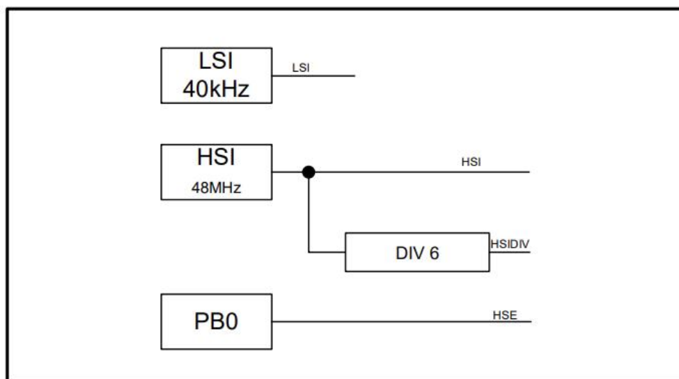
图 6.6 系统时钟源
