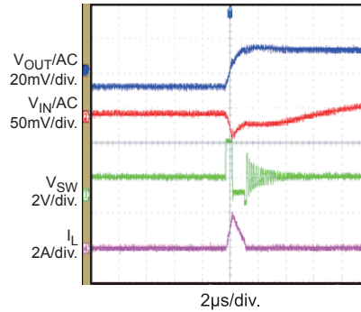
Input/Output Ripple
