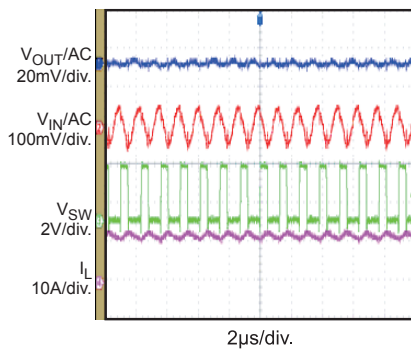
Input/Output Ripple
