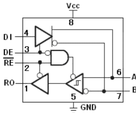
图2: MAX485CSA 逻辑图
