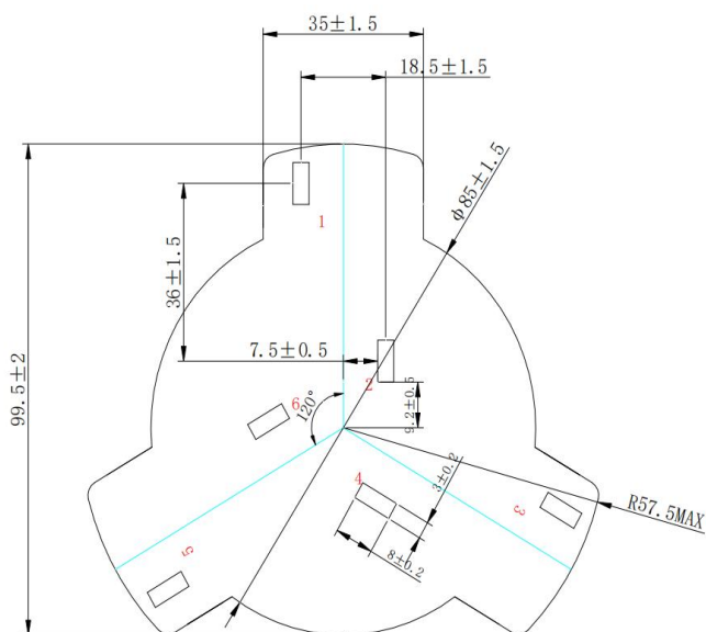
底视图
