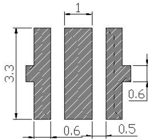
焊盘建议图
