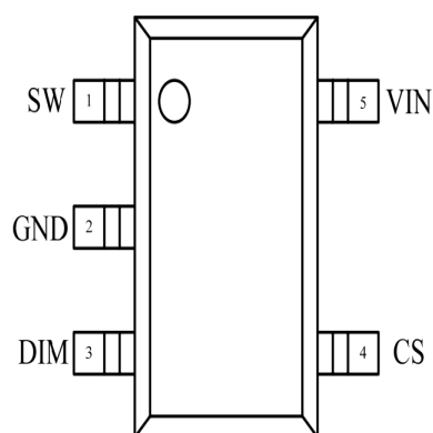
SOT23-5
