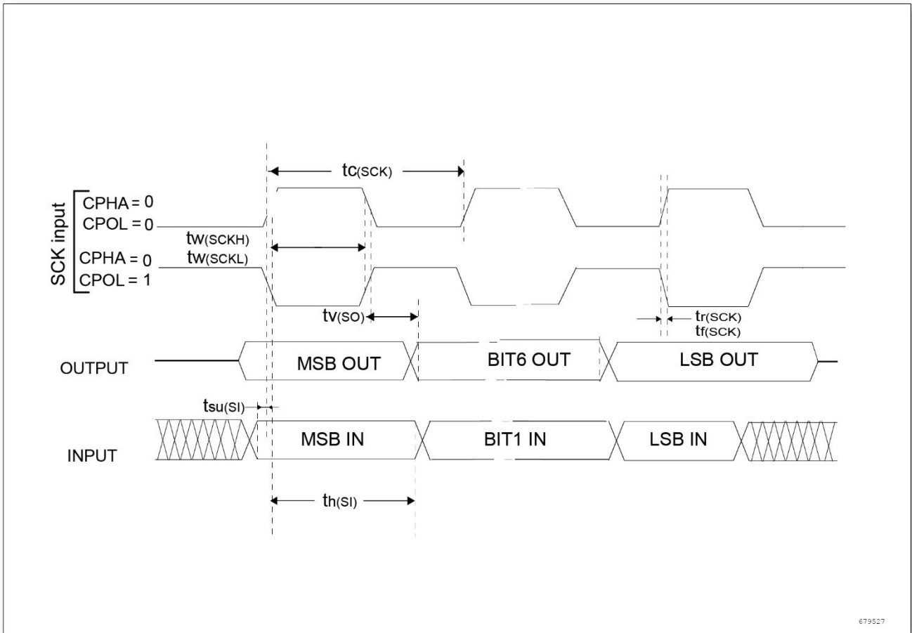
图 18 USART 同步模式时序图
