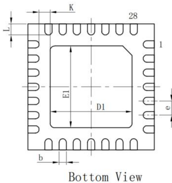
QFN28 4*4, 封装尺寸 POD 图,
