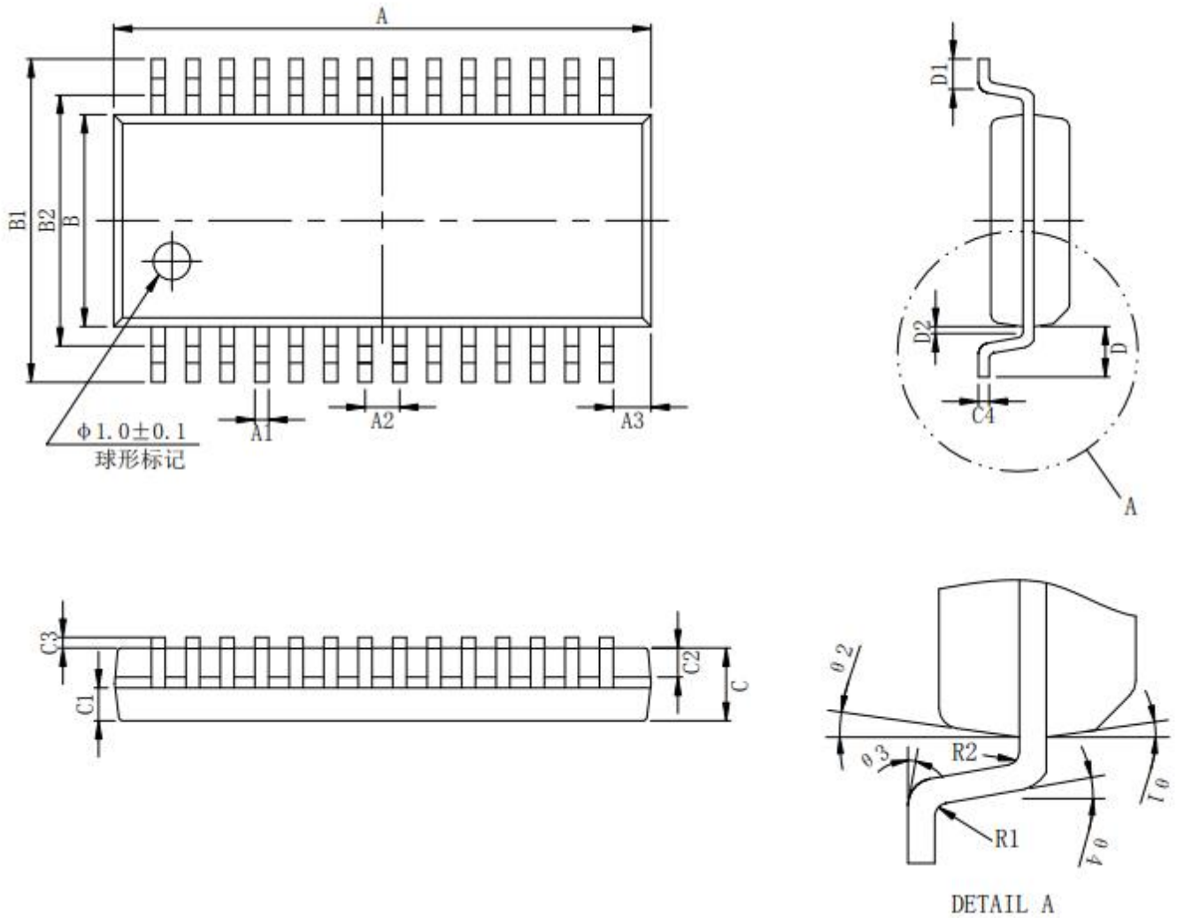
SSOP28 9.8*3.85, 封装尺寸 POD 图 单位:mm
