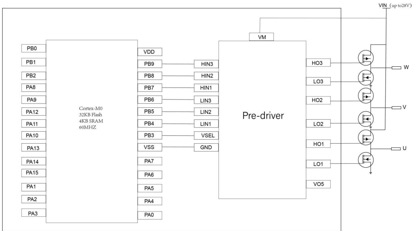
图 10 功能框图与应用参考电路
