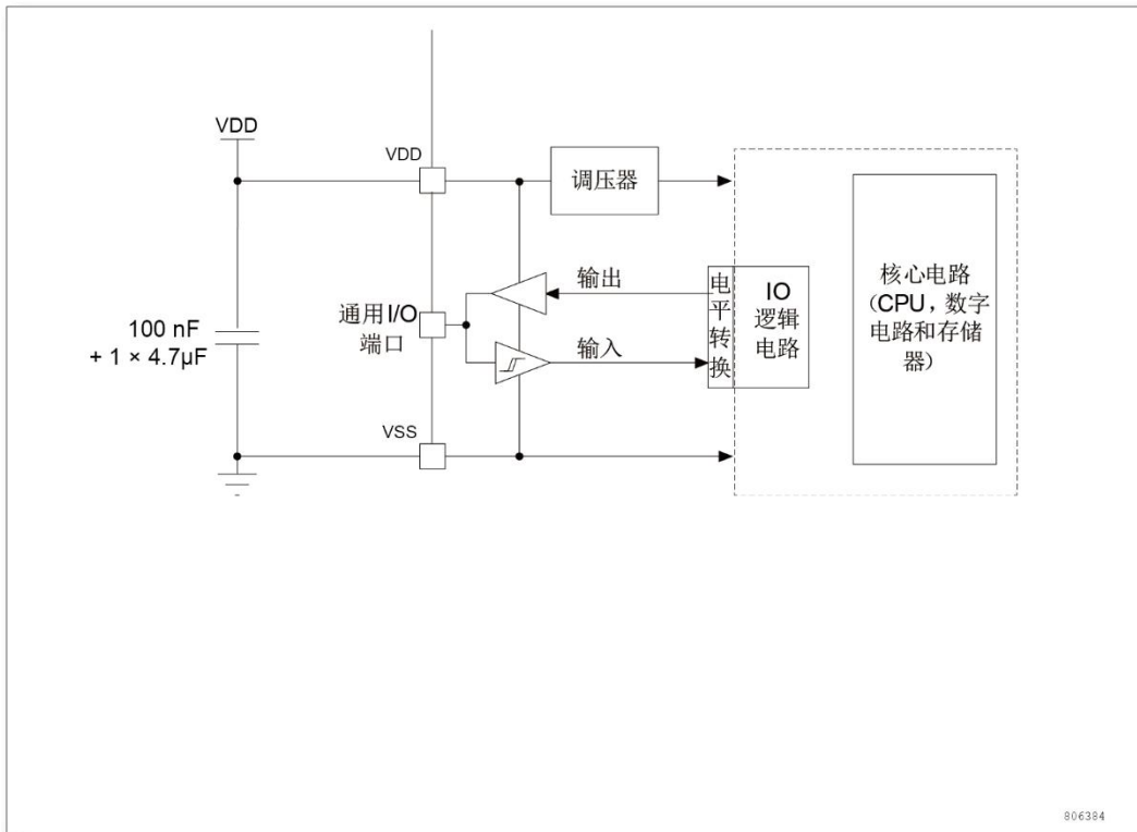
图 13 供电方案
