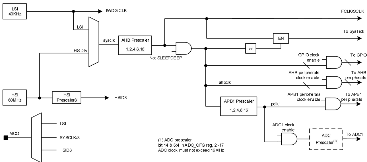
图 3 时钟树
