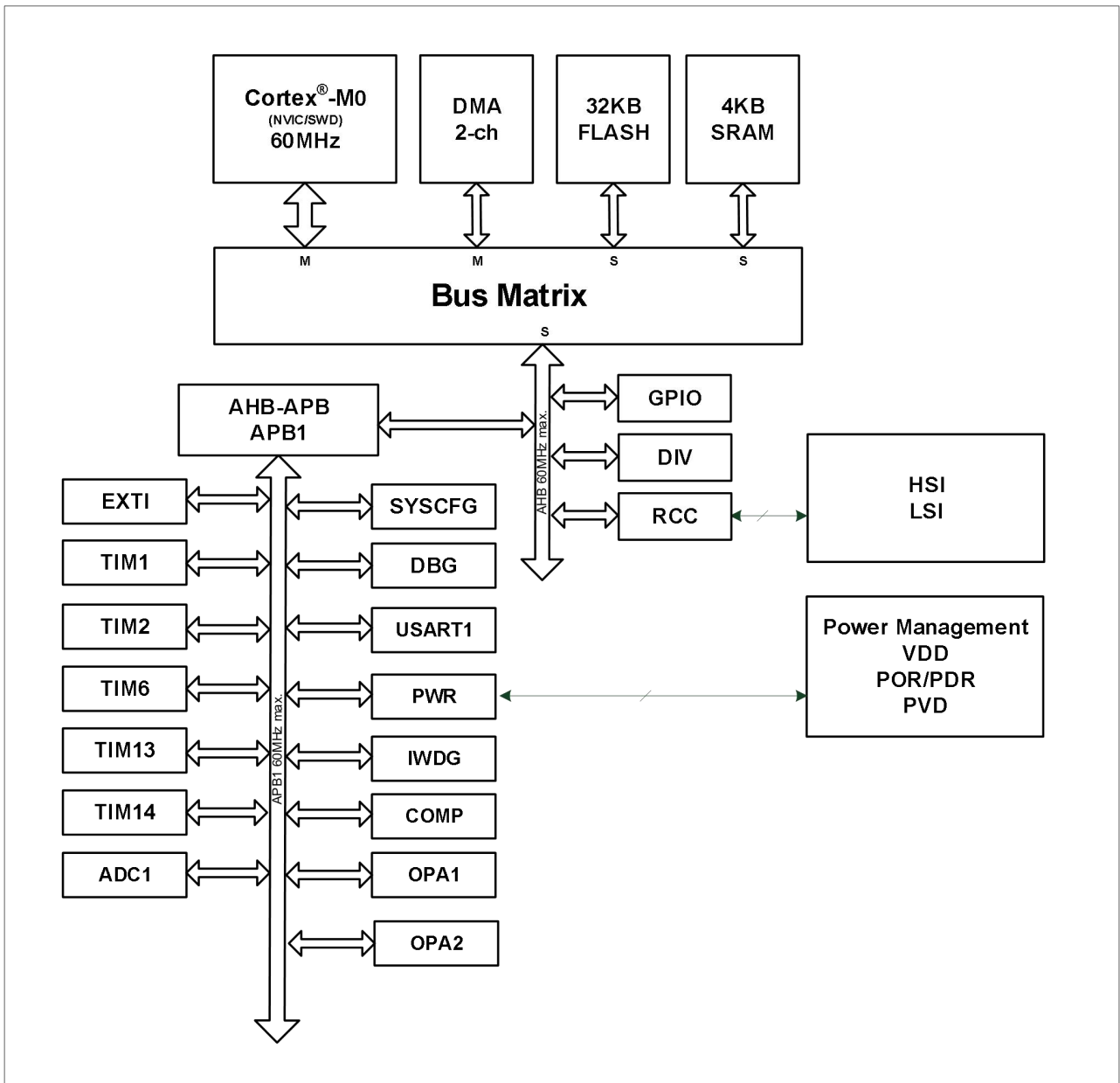
图 2 模块框图
