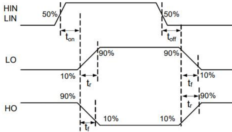
图 26 开关时序
