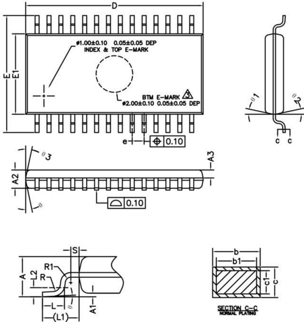
TSSOP28 9.6*4.3, 封装尺寸 POD 图,
