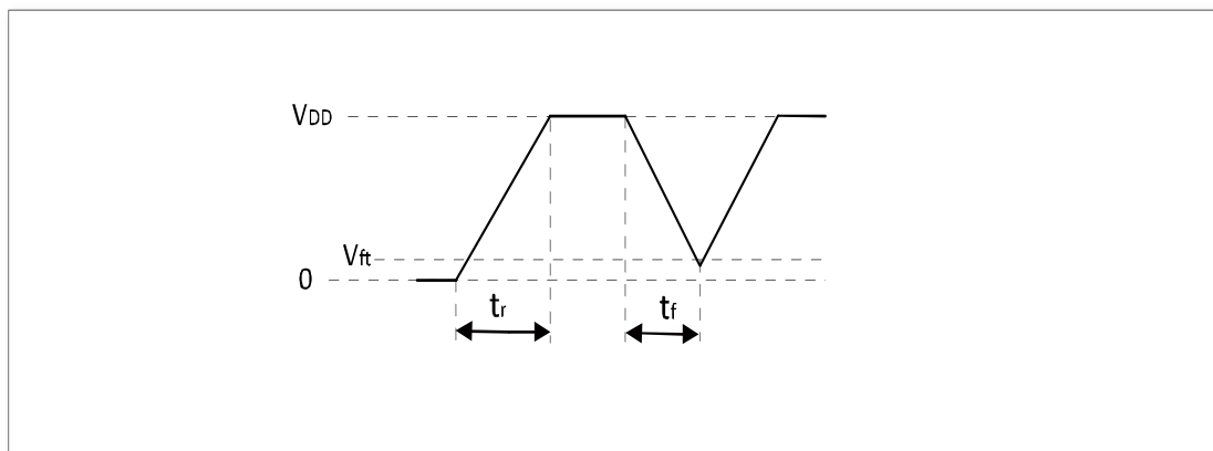
图 15 上电与掉电波形
