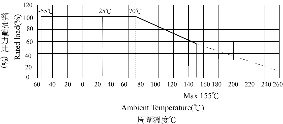
圖一 電力遞減曲線 Figure 1 Power derating curve 線繞型水泥電阻 Wire Wound Cement Type
