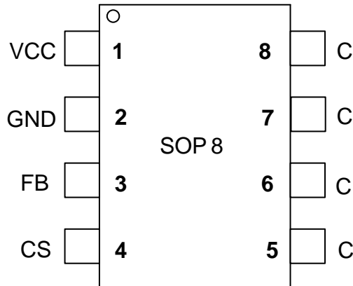
图 2 管脚封装图
