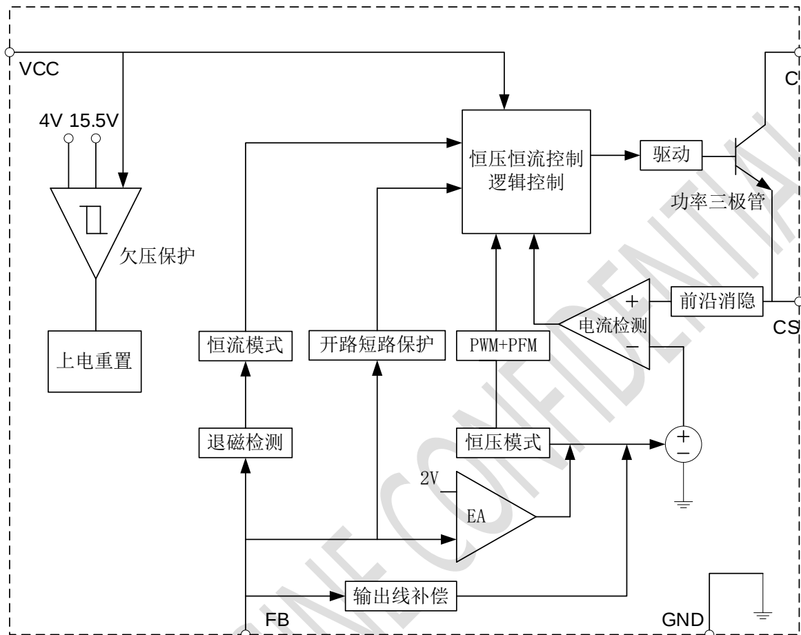
图3 SZ3702X 内部框图
