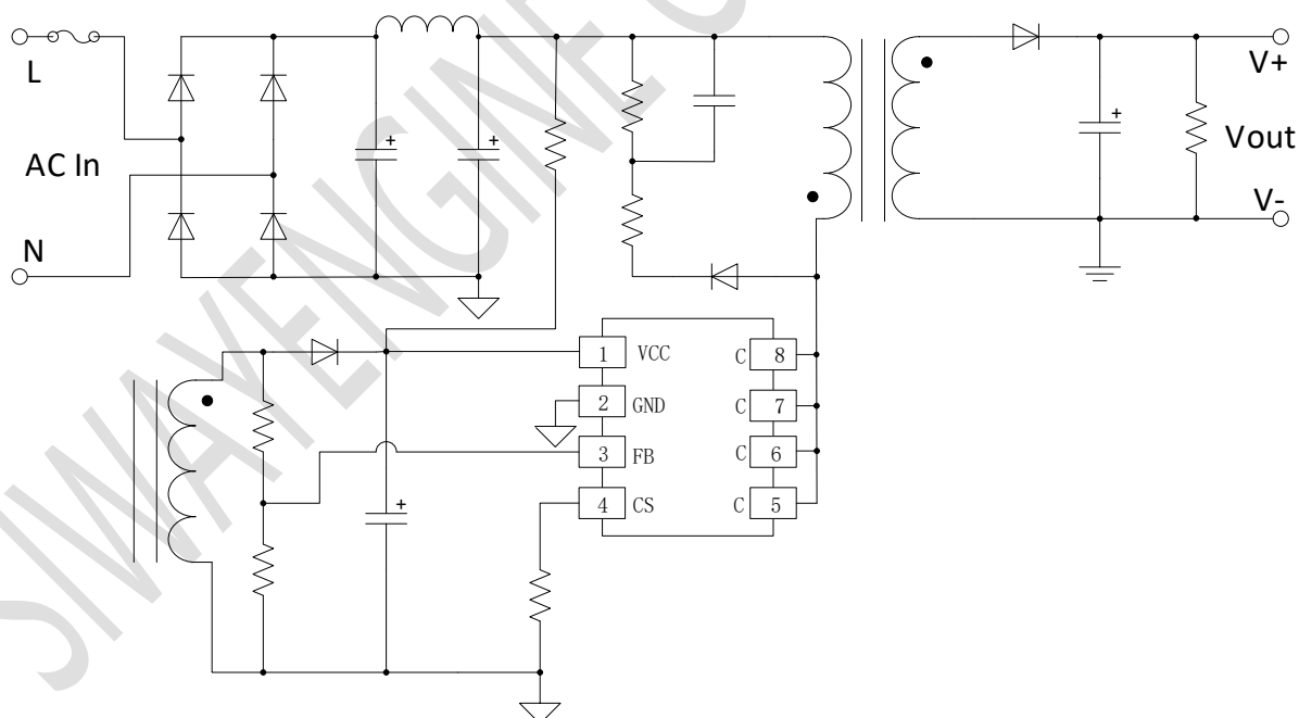
图 1 SZ3702X 典型应用图
