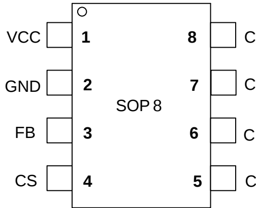
图 2 管脚封装图
