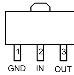
SOT89-3 (L type, SK6513ST3B)
