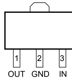
SOT89-3 (SK6513ST3A)
