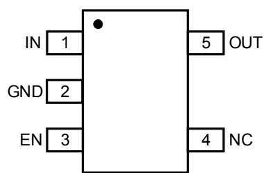
SOT23-5 (SK6513SS5E)
