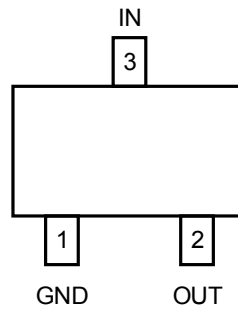
SOT23-3 (SK6513SS3)
