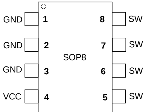
图 2 管脚封装图
