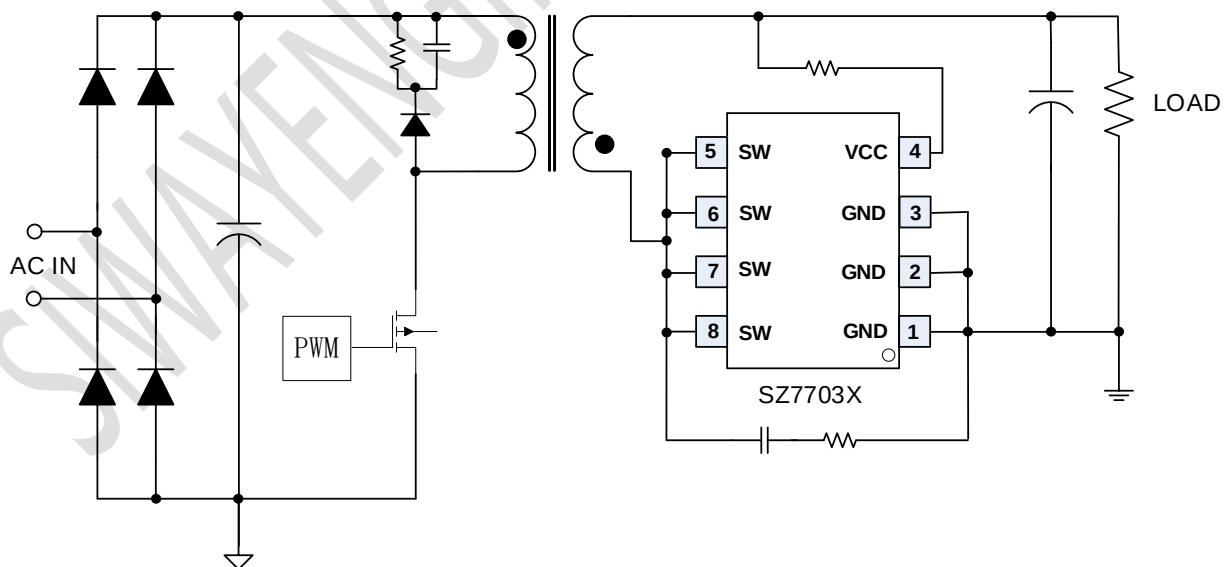
图 1 SZ7703X 典型应用电路
