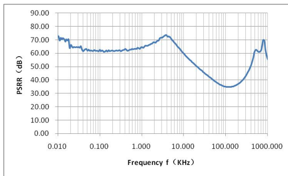
PSRR
