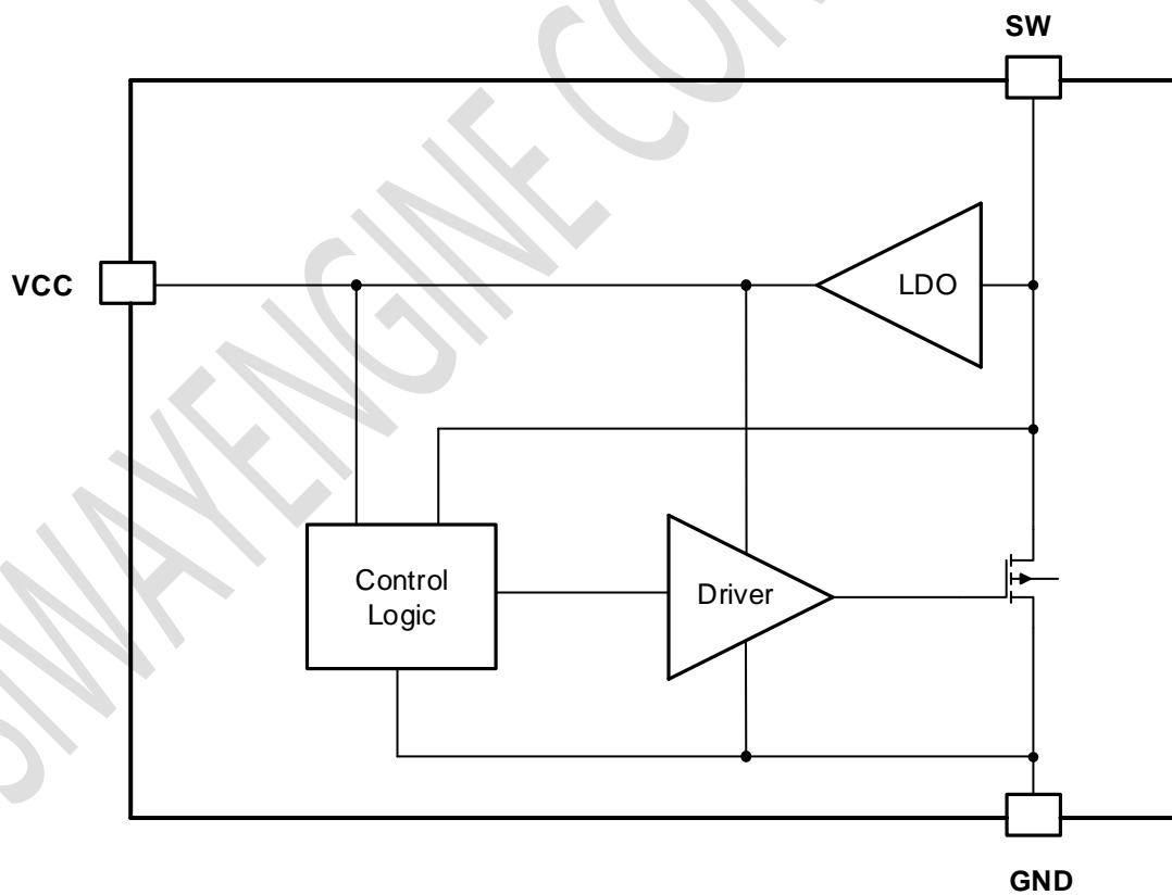
图 3 SZ7020BA 内部框图
