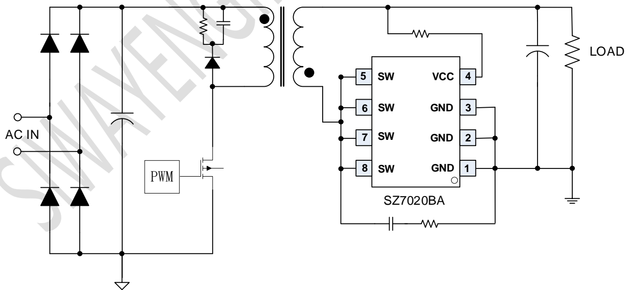
图 1 SZ7020BA 典型应用电路
