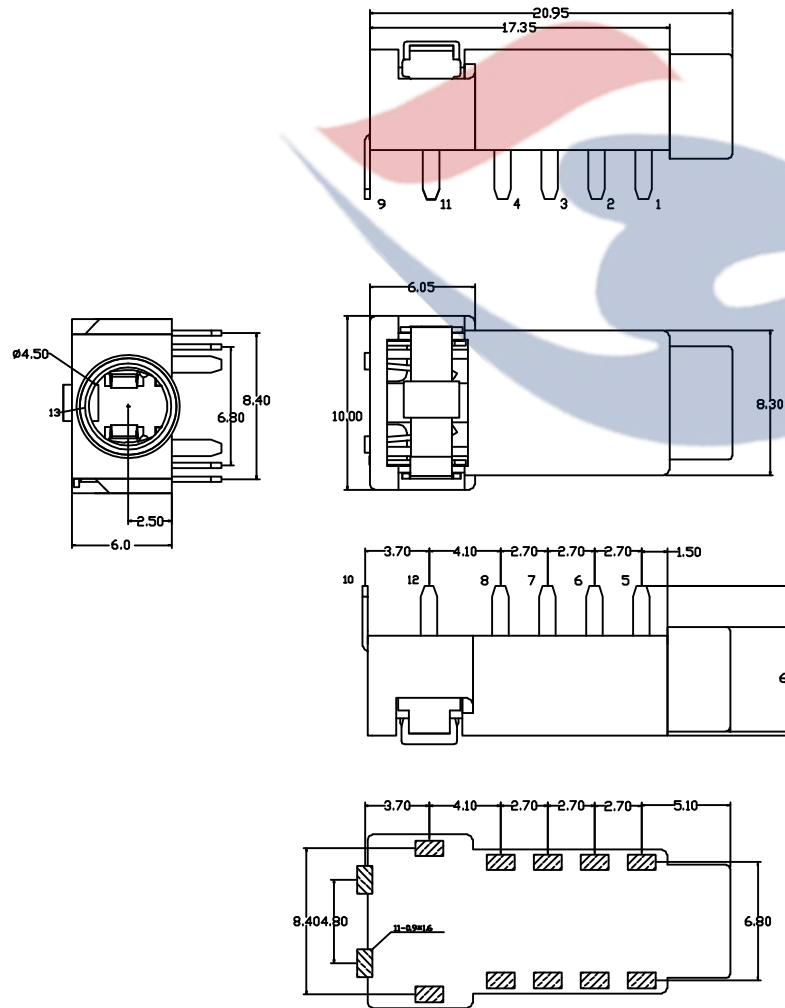
P.C.B LAYOUT
