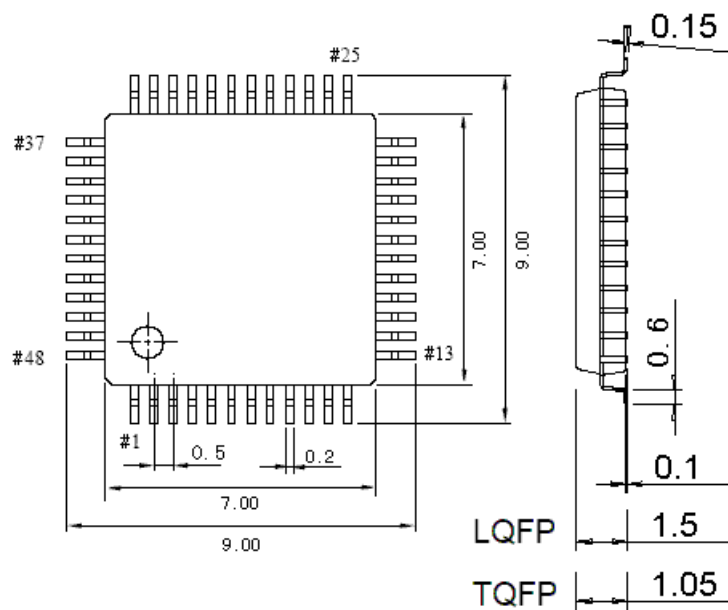
图 4-2 LQFP48 封装
