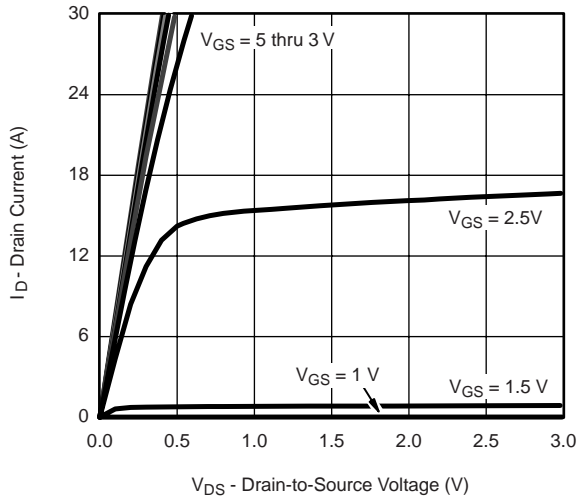
V_{GS} = 1\text{ V} V_{GS} = 1.5\text{ V} V_{GS} = 2.5\text{ V} V_{GS} = 5\text{ thru }3\text{ V} Output Characteristics
