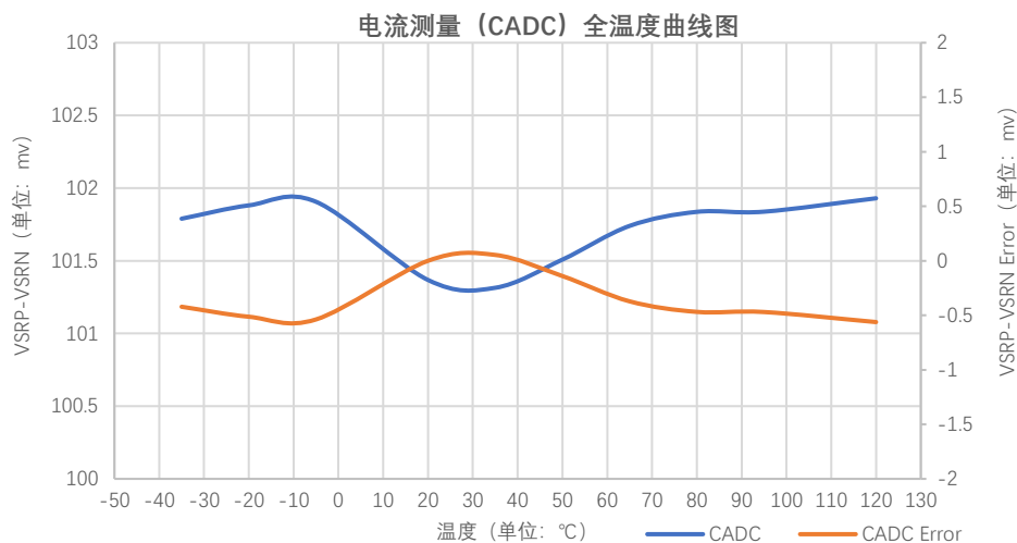
图 8.2 CADC 电流典型测量温度曲线
