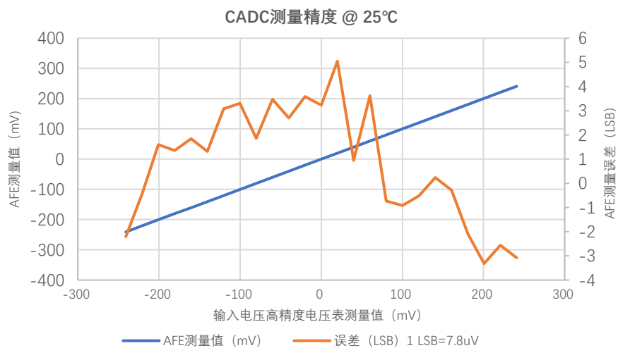
图 8.1 CADC 电流典型测量误差
