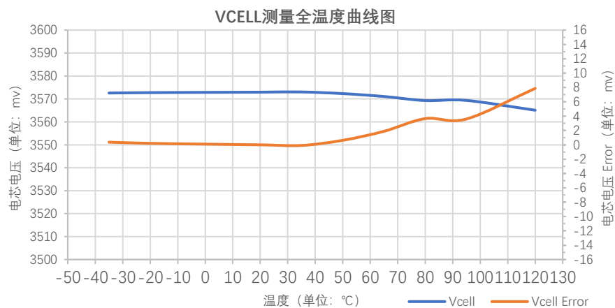
图 8.3 CELL 电压典型测量温度曲线
