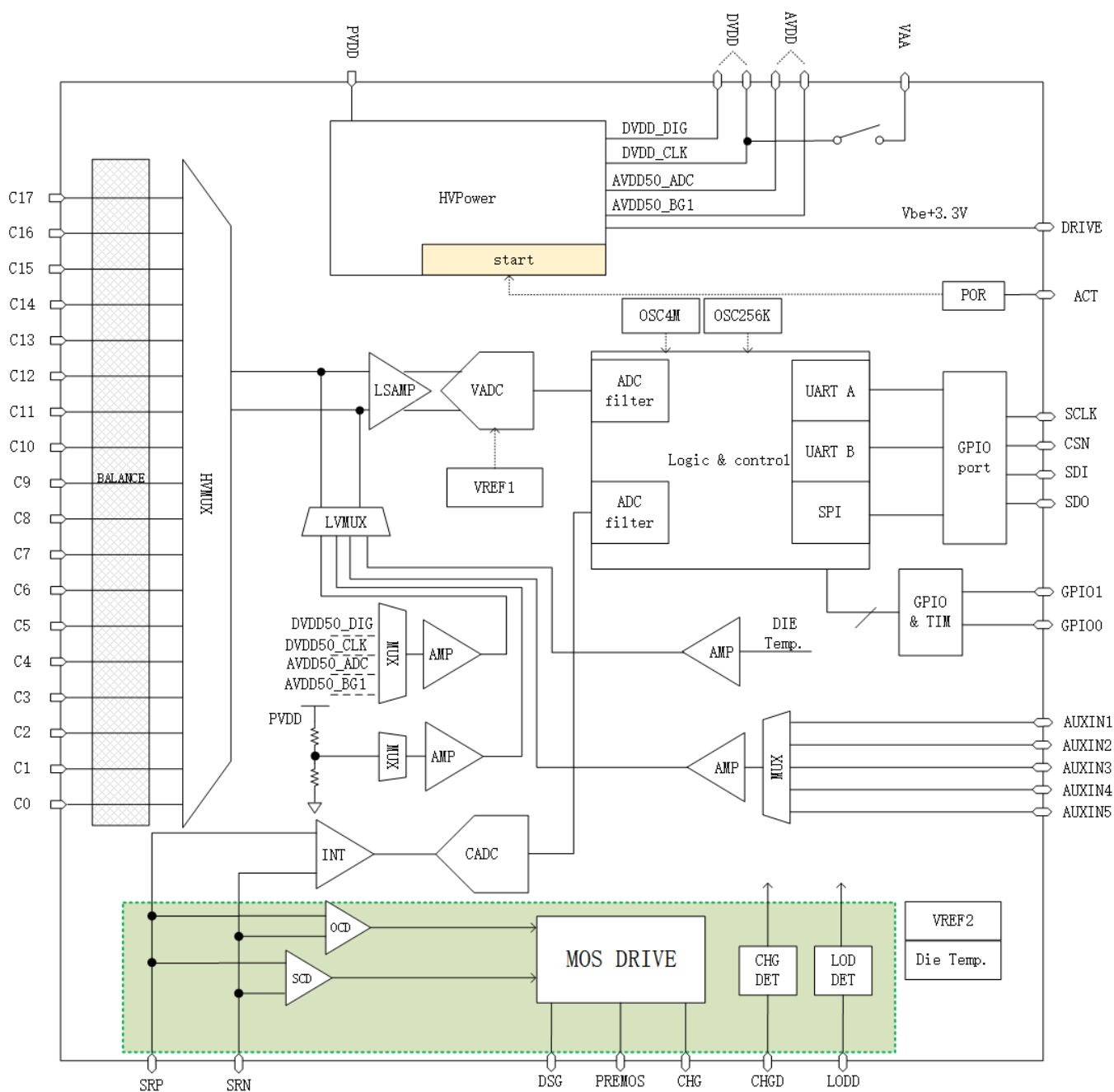
图 6 内部框图
