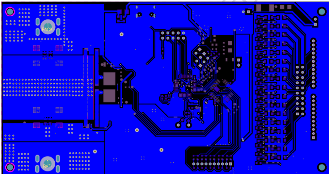
图 12.6.2 应用板（160mmX86mm）底层布线示例
