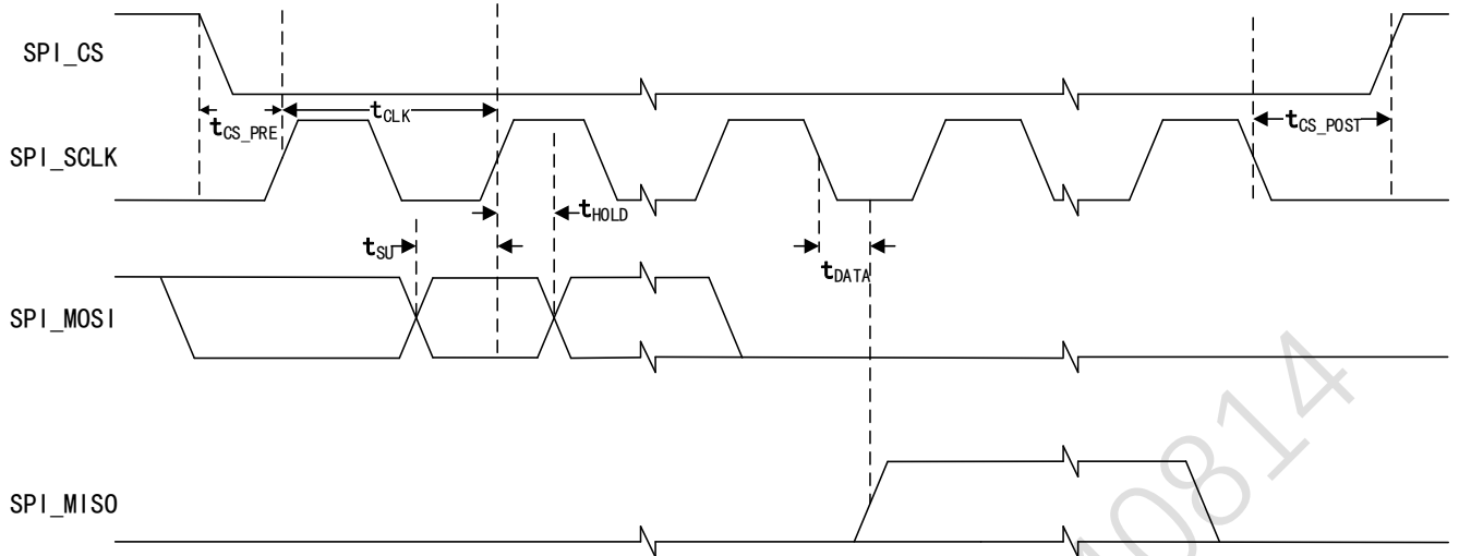
图 7.3 SPI 时序图
