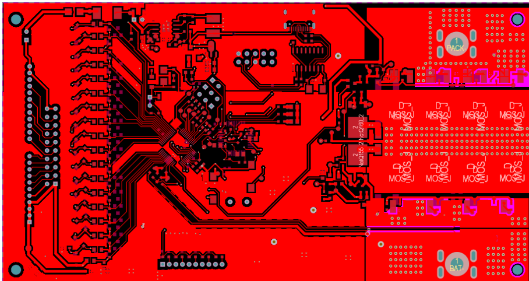
图 12.6.1 应用板（160mmX86mm）顶层布线示例
