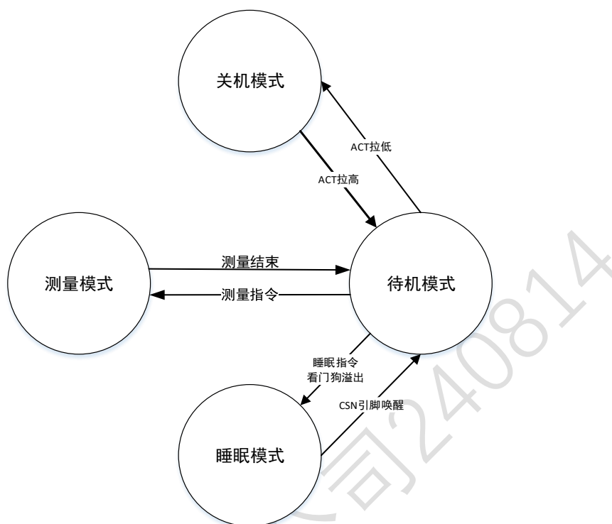
图 9 工作模式
