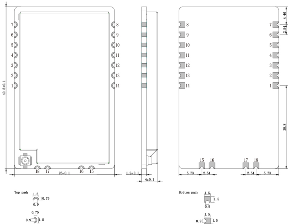
图 10 推荐封装
