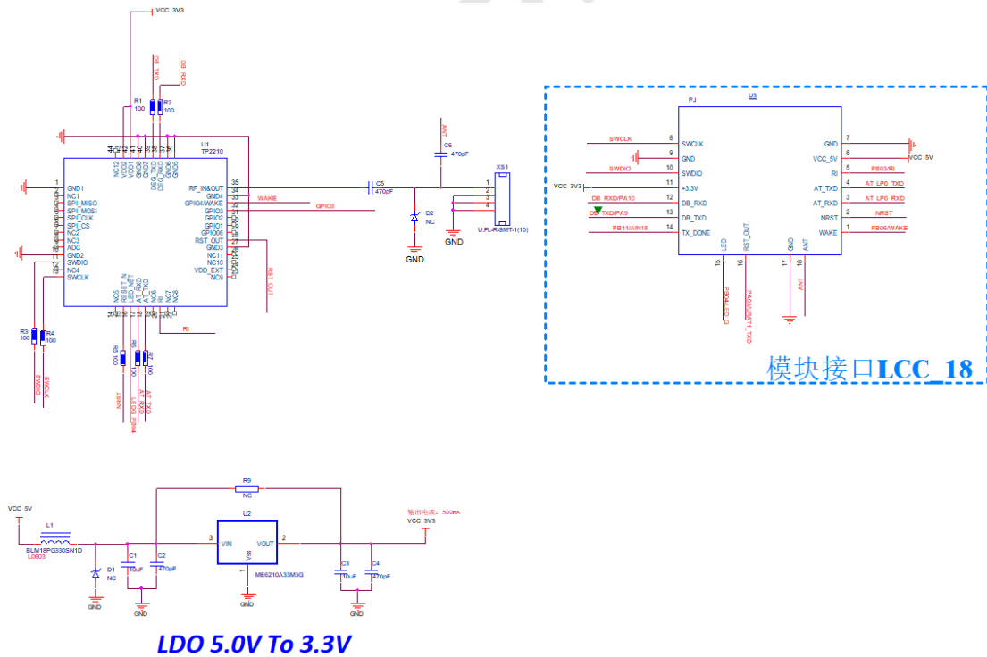
图 6 参考原理图
