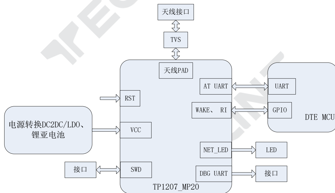
图 5 模块外围电路框架
