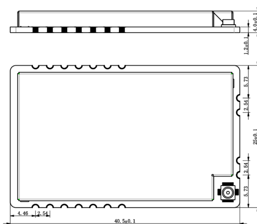
图 9 俯视及侧视尺寸图
