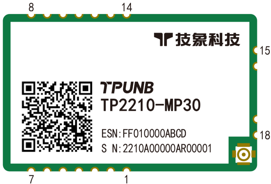
图 4 模块引脚图
