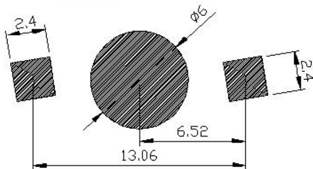
焊盘建议图
