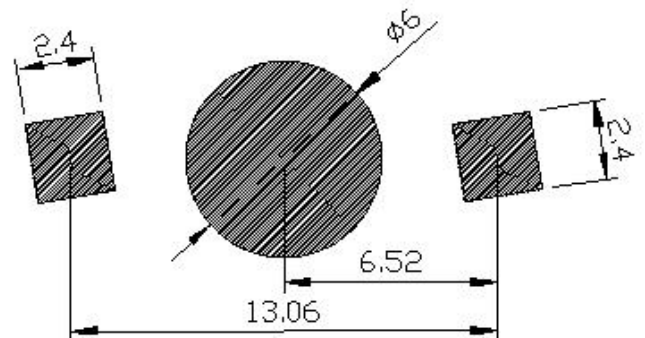
焊盘建议图
