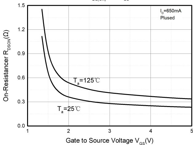
R_{DS(ON)} - V_{GS}
