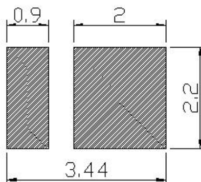
焊盘建议图
