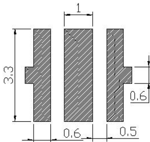
焊盘建议图
