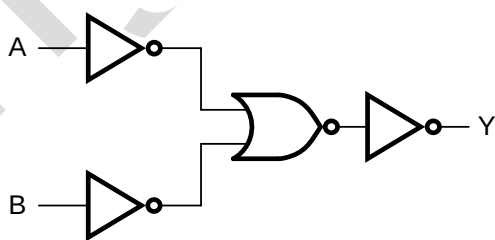
图 3 逻辑框图
