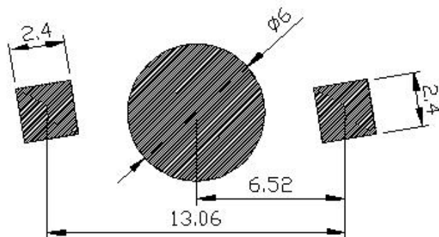
焊盘建议图
