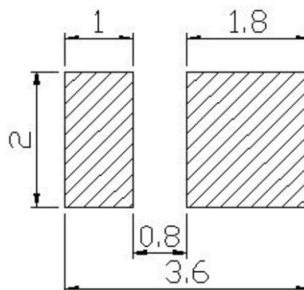
焊盘建议图
